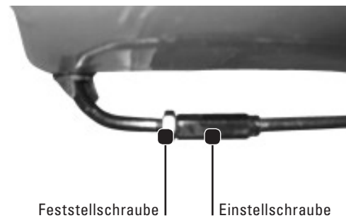
Feststellschraube
